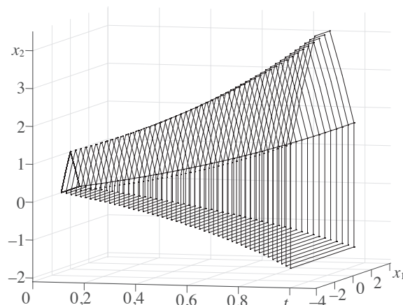
Рис. 5. Розв'язок X(t) диференціального рівняння (2) з похідною Хукухарі на проміжку [0, 1] .
