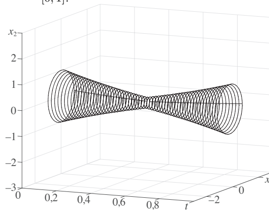
Рис. 12. Мішаний розв'язок Y_2(t) диференціального рівняння (7) із PS- і VG-похідною на проміжку [0, 1] .
