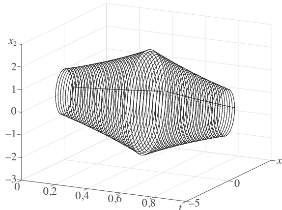
Рис. 11. Мішаний розв'язок Y_1(t) диференціального рівняння (7) із PS- і VG-похідною на проміжку [0, 1] .
