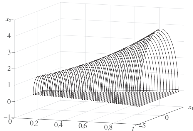
Рис. 17. Перший базовий розв'язок X_1(t) диференціального рівняння (16) із PS-похідною та диференціального рівняння (17) із BG-похідною на проміжку [0, 1] .
