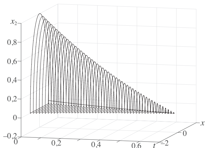
Рис. 22. Другий базовий розв'язок X_2(t) диференціального рівняння (26) із BG-похідною на проміжку [0, \ln(2)] .
