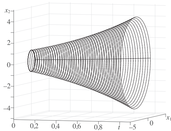
Рис. 9. Перший базовий розв'язок X_1(t) диференціального рівняння (7) із PS- і VG-похідною на проміжку [0, 1] .
