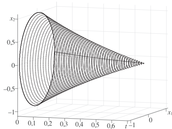
Рис. 10. Другий базовий розв'язок X_2(t) диференціального рівняння (7) з PS- і VG-похідною на проміжку [0, \ln(2)] .
